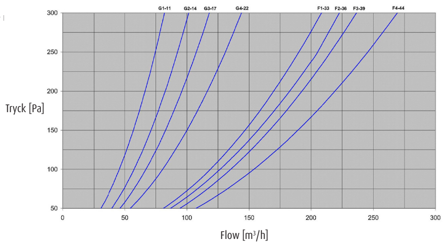
Innjusteringsdiagram
