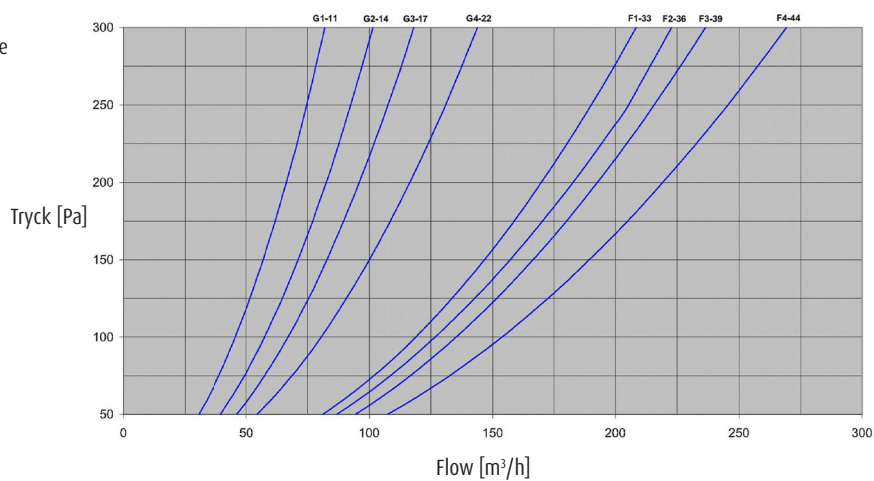
Innjusteringsdiagram
